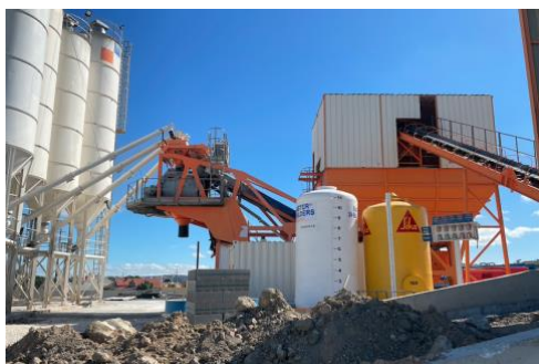
Figura 3 - zona produção betão
